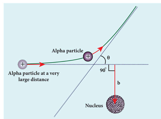
Figure 9.12 Impact parameter
